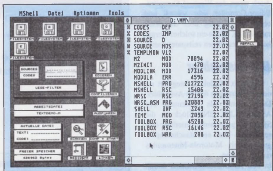
Bild 2: Die Shell
