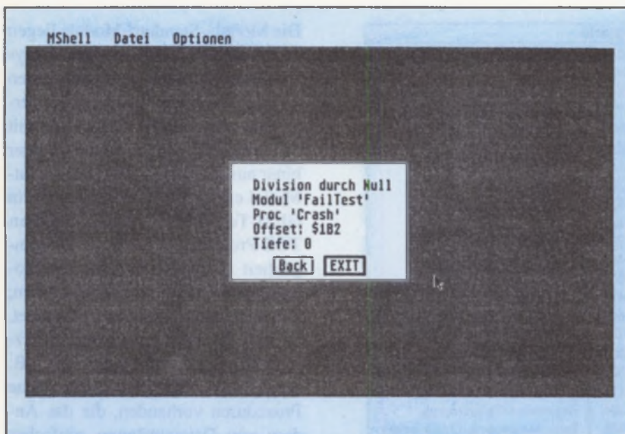
Bild 6: Ein Laufzeitfehler ...
