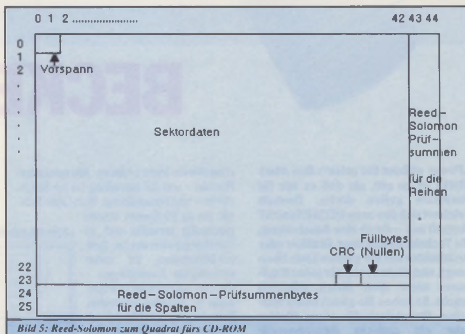
Bild 5: Reed-Solomon zum Quadrat fürs CD-ROM
