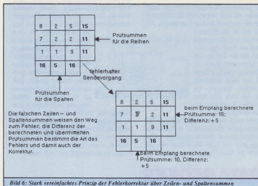
Bild 6: Stark vereinfachtes Prinzip der Fehlerkorrektur über Zeilen- und Spaltensummen
