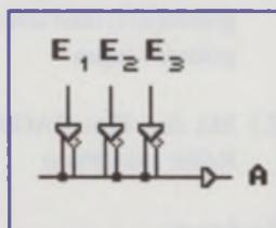
Bild 4: UND-Term: E1^*/E2 \cdot E3
