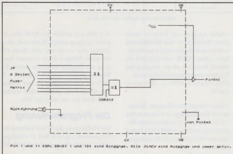
Bild 8: 'normaler' Ausgang (SYN = 1, AC0 = 0, AC1(n) = 0)
