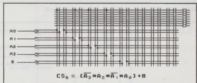
Bild 5: Unser Beispiel im GAL.
