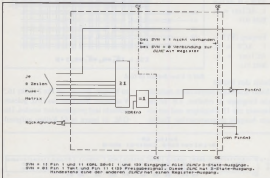
Bild 9: 3-State-Ausgang mit Freigabe und Rückführung (SYN = 0 oder 1, AC0 = 1, AC1(n) = 1)
