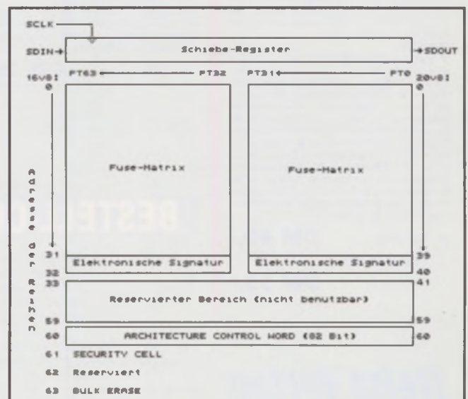
Bild 13: Interne Organisation
