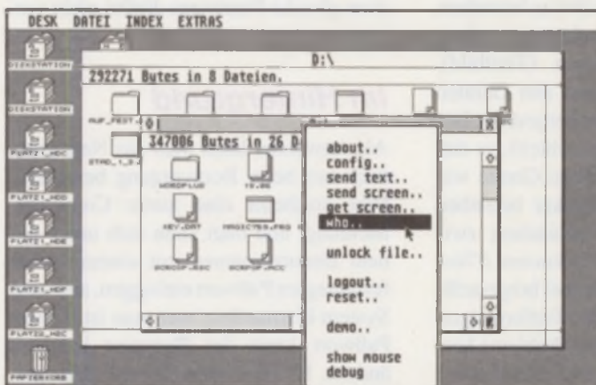
Bild 2: Das Popup-Accessory
