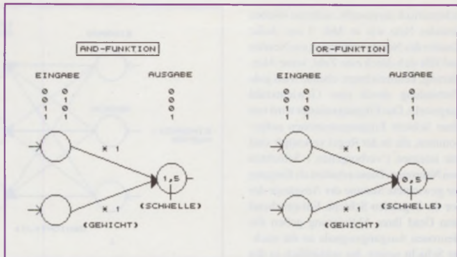
Abb. 4: Neuronales Netz für AND- und OR-Funktion
