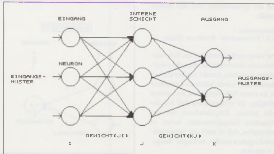
Abb. 3: Neutrales Netz mit Vorwärtsausbreitung
