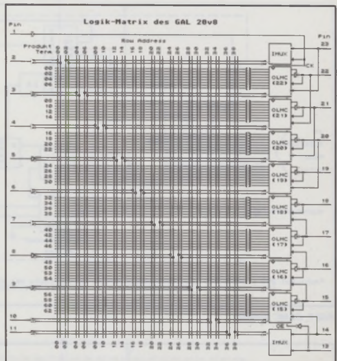
Bild 3: Interner Aufbau des GAL 20v8
