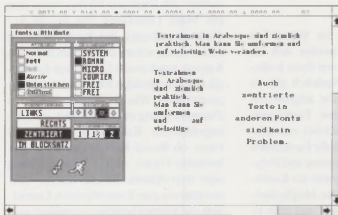
Bild 3: Vektortextfunktion
