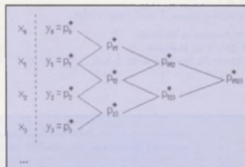
Bild 6: Das Schema von Neville
