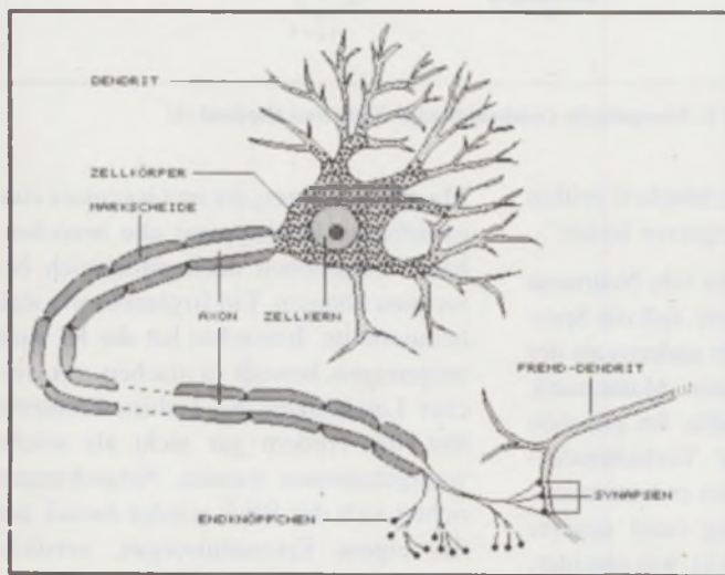
Abb. 2: Nervenzelle
