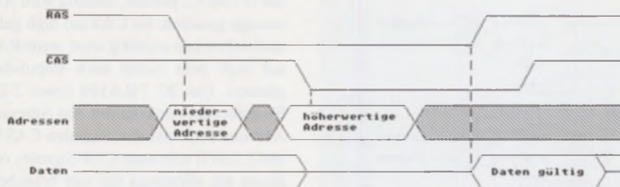
Bild 2: Das Impulsdiagramm
