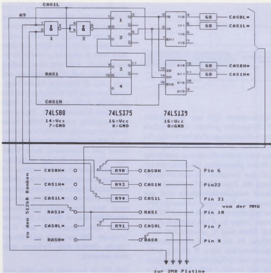
Bild 1: Das Schaltbild
