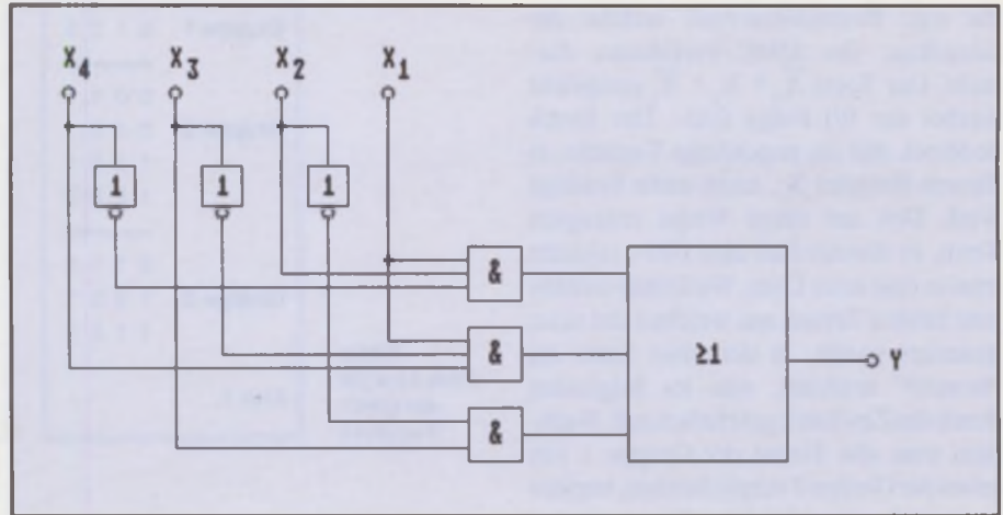
Bild 8: Die optimierte Schaltung nach Glg. (4) zeigt eine beträchtliche Einsparung an Schaltelementen.
