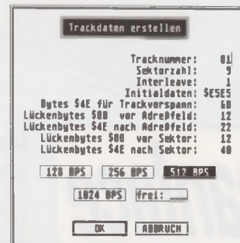
Bild 5: Besonders für das Neuformatieren eines Tracks sind viele Manipulationen denkbar.
