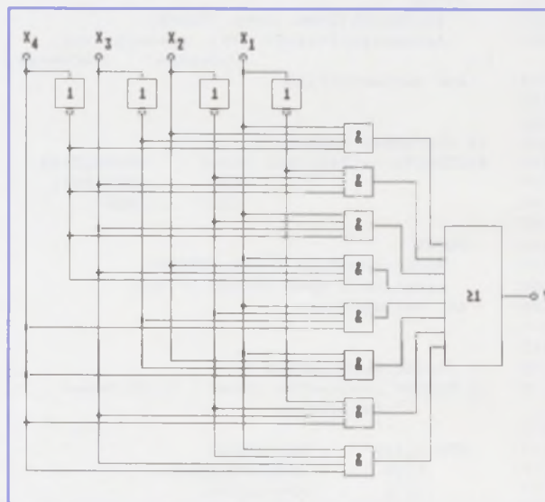
Bild 2: Schaltungsrealisierung der Wertetafel aus Bild 1 mittels disjunktiver Normalform
