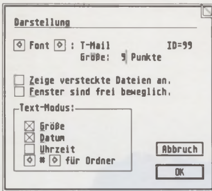
Bild 1: Eine Dialogbox aus der GEMINI-Shell
