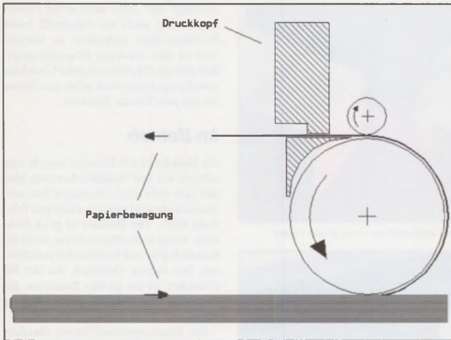
So läuft Papier durch den Deskjet PLUS.
