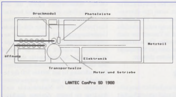
Abb. 2: Verbindungsplan
