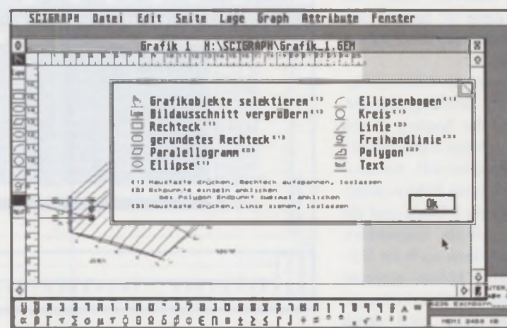
Bild 7: Eine Hilftafel wurde einge- blendet. Sie bezieht sich immer auf eine vorher ausge- wählte Funktion.
