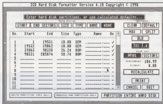
Bild 4: Teile und herrsche über 1000 Knöpfe
