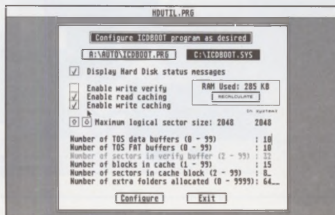
Bild 5: Der ICD-Plattentreiber zeigt sich wandlungsfähig
