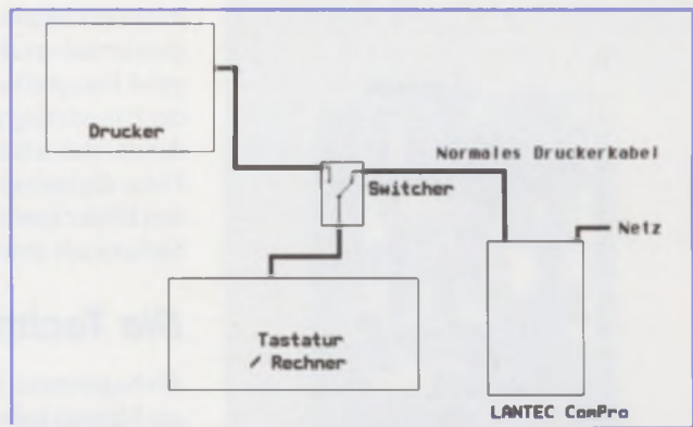
Abb. 3: Ein Switcher sorgt für wahlweisen Drucker- oder Scannerbetrieb.
