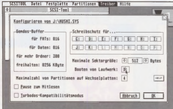
Bild 6: Diese Treiber- Parameter lassen sich verändern
