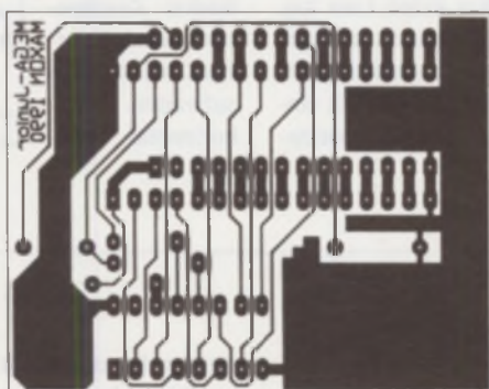
Mega-Adapter Lötseite
