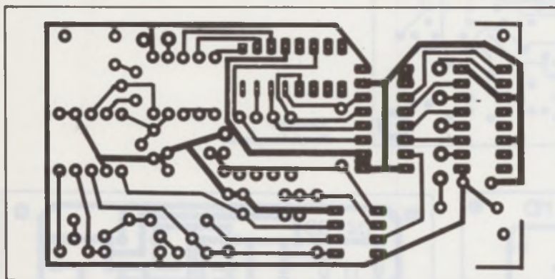
Scanner Lötseite
