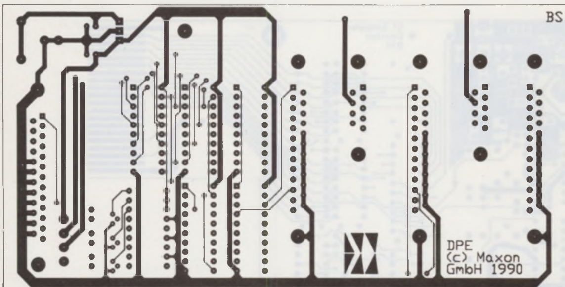
DPE Bestückungsseite
