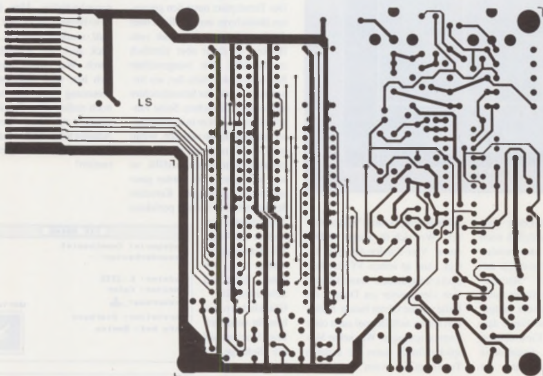
Easytizer Lötseite
