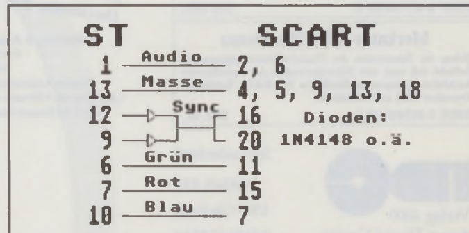
Bild 1: Verbindung ST-Monitorbuchse - SCART-Stecker
