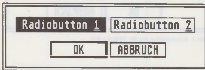
Abb. 1: Beispieldialog
