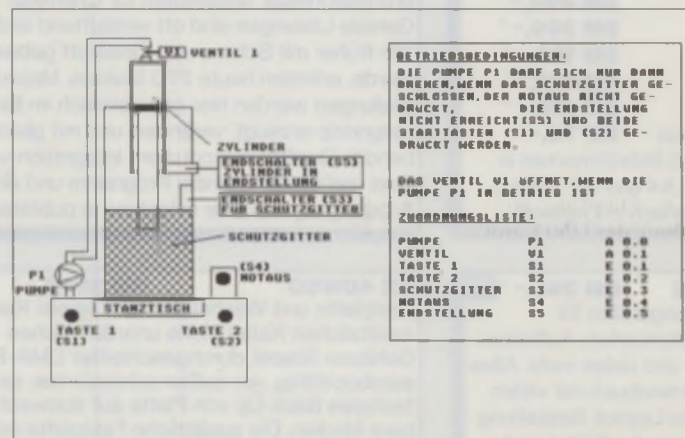
Bild 4: Steuerung einer Stanzmaschine
