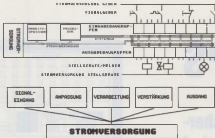
Bild 2: Übersicht über den Grundaufbau eines SPS-Gerätes
