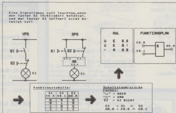
Bild 3: Umsetzung Stromlaufplan/ AWL
