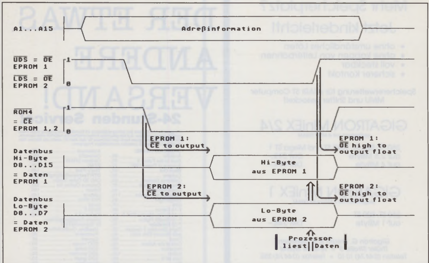
Bild 8a: Das Lese-Timing einer 16-Bit-EPROM-Karte am ROM-Port
