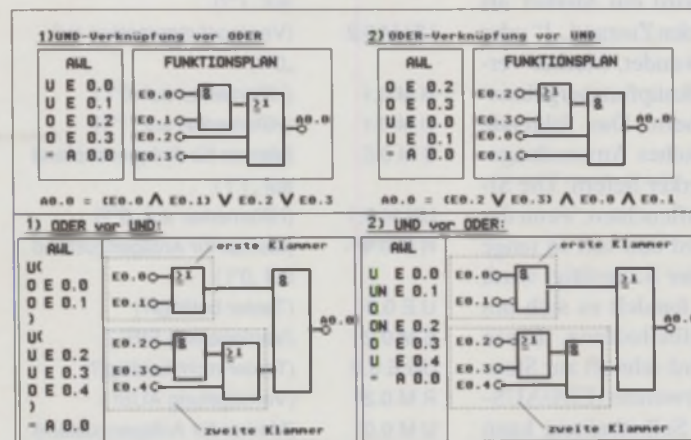
Bild 6: Logische Verknüpfung bei der SPS-Programmierung
