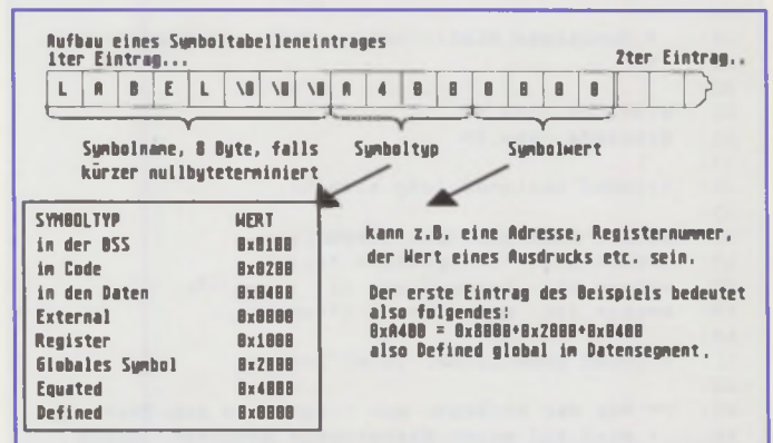
Bild 2: Der Aufbau eines Symboltabelleintrags
