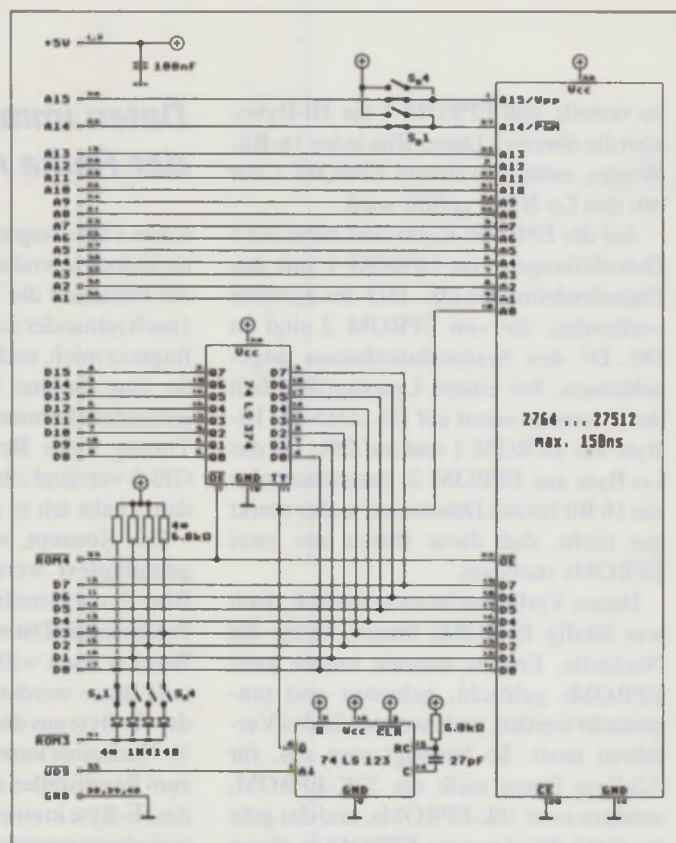
Bild 3: Im Schaltplan sieht man, wie die acht zusätzlichen Datenleitungen gewonnen werden.
