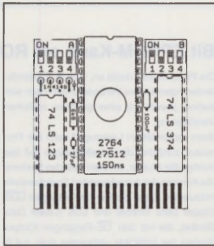
Bild 4: Die enge Bestückung der Platine erfordert
