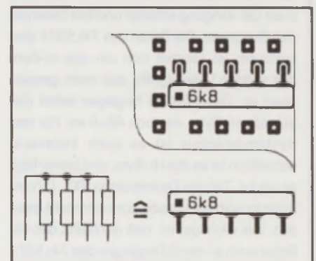
Bild 6: Das SIL-Array wird auf der Platinenunterseite auf fünf Kontaktflächen aufgelötet.
