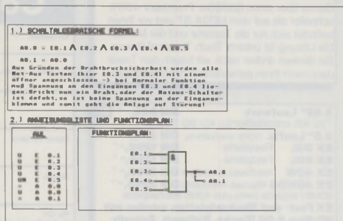
Bild 5: Erstellung der AWL zu dieser Steuerung
