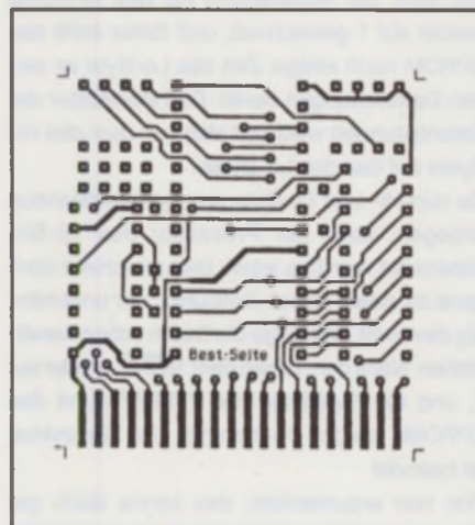
Bild 5b: Platinen-Layout - Bestückungsseite
