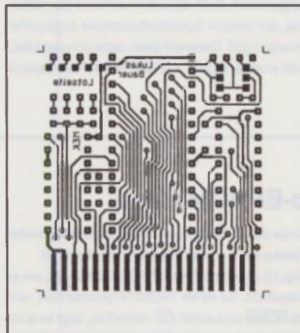
Bild 5a: Platinen-Layout - Lötseite
