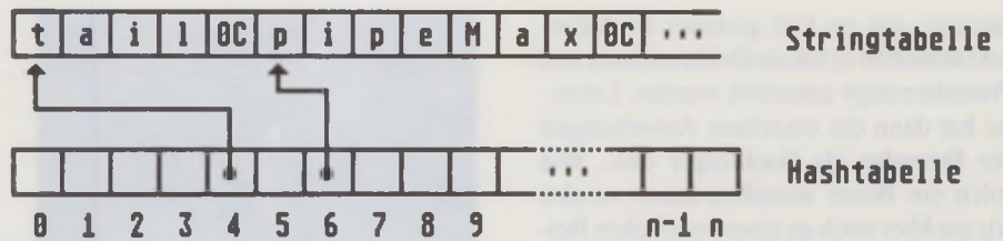
Abb. 2: Beispiel einer Bezeichnertabelle
