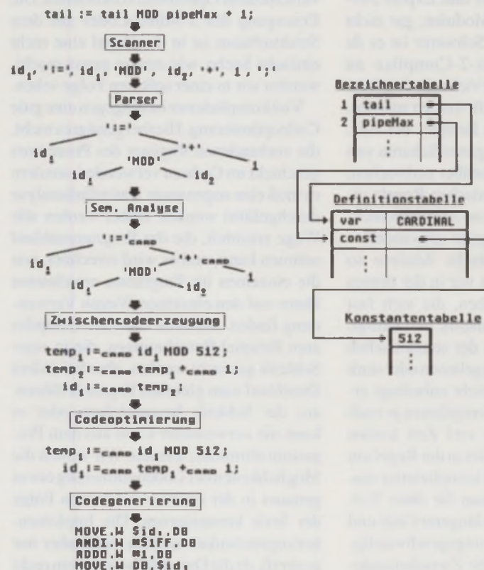
Abb. 3: Transformation eines arithmetischen Ausdrucks
