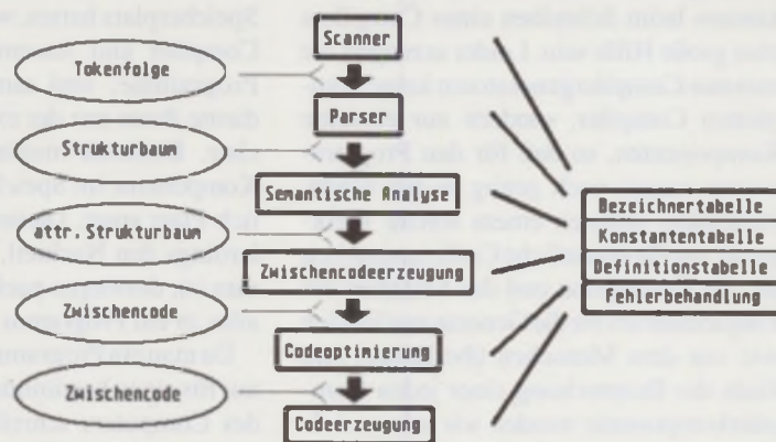
Abb. 1: Die Phasen eines Compilers und die von ihnen erzeugten Zwischenformen
