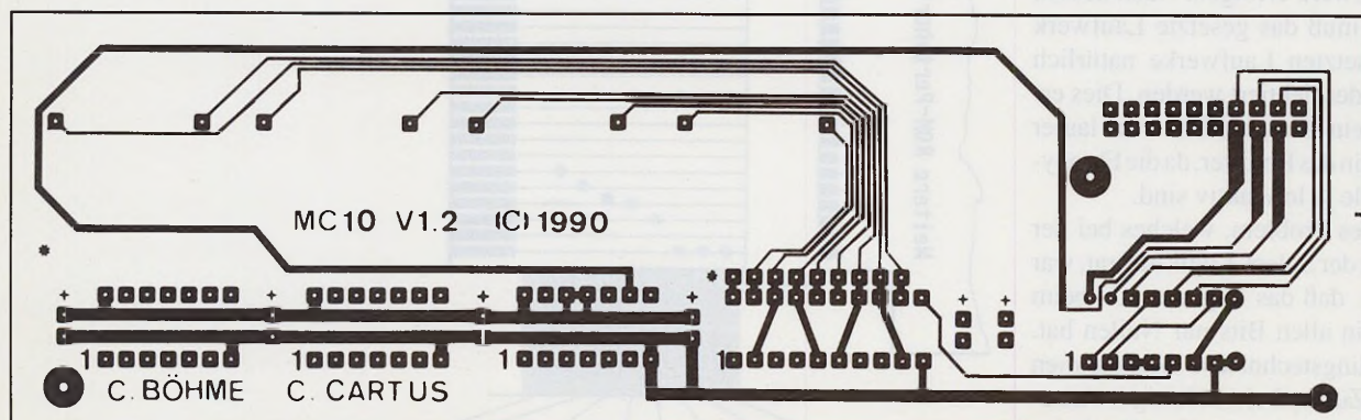
Bild 18: Die Platinenoberseite von MC10
