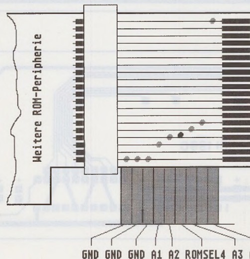
Bild 13: Der Flachbandleistungsanschlus an der ROM-Port-Verlängerung
