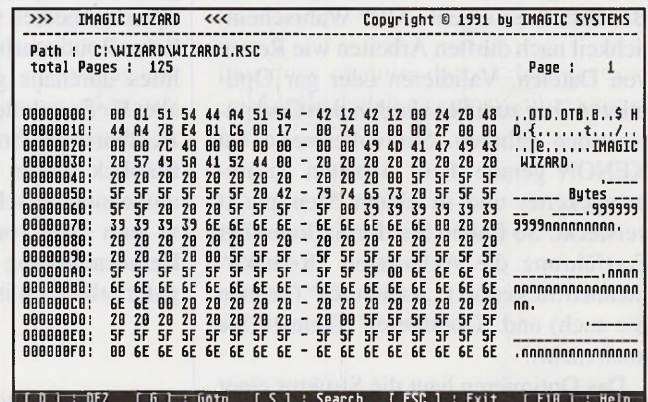
Bild 2: So präsentiert sich uns der Disketteneditor
