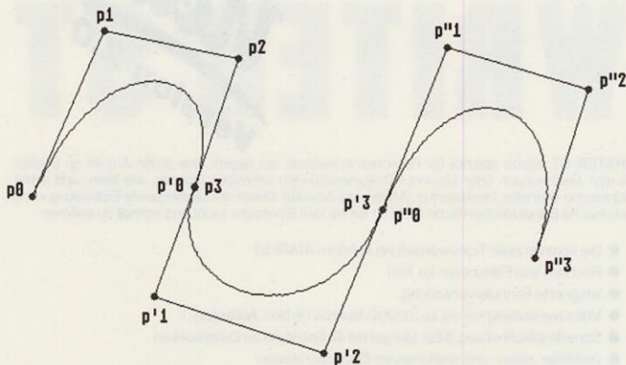
Abb.4: Drei zusammengesetzte Bézierkurven mit glatten Übergängen
