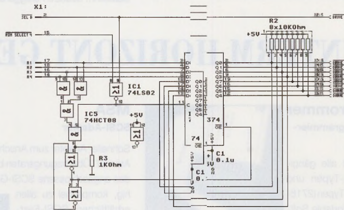
Bild 7: Die Selektierungslogik von MC10
