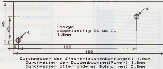
Bild 10: Die mechanischen Grundmaße der MC10-Hauptplatine
