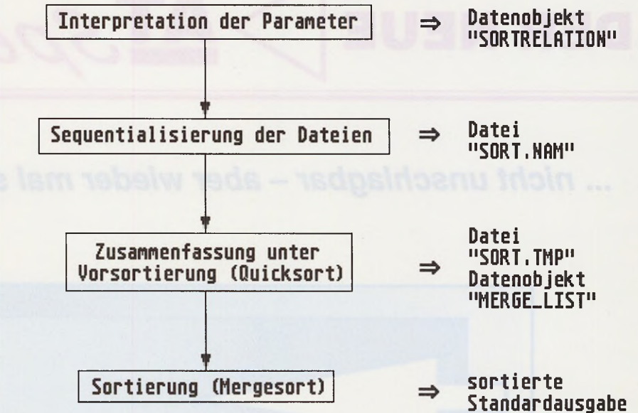
Bild 1: Die Sortierphasen des Kommandos SORT
