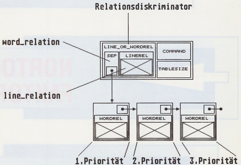
Bild 2: Darstellung des Datentyps SORTRELATION
