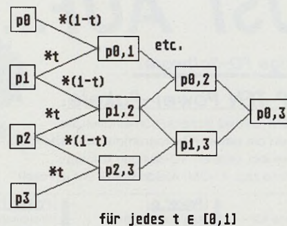
Abb.5: Numerische Berechnung von Bézierkurven
