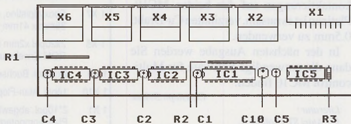
Bild 12: Der Bestückungsplan des MC10
