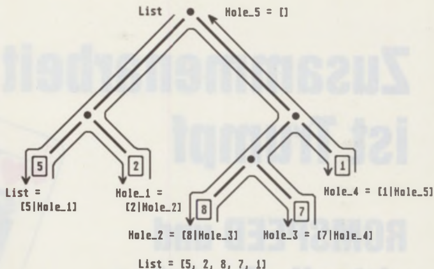
Abb. 4: Linearisierung eines Binärbaums mit Differenzlisten
