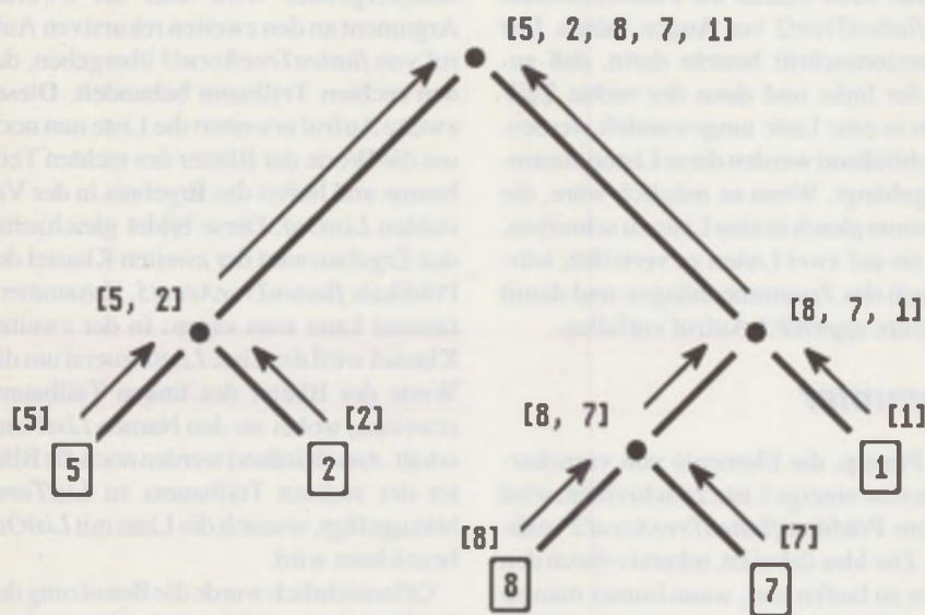
Abb. 2: Naive Linearisierung eines Binärbaums
