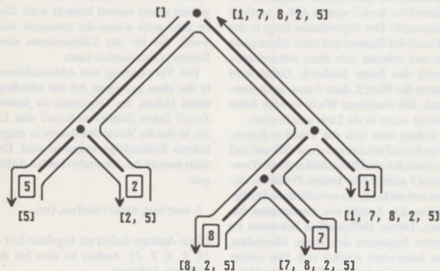
Abb. 3: Linearisierung eines Binärbaums mit einem Akkumulator
