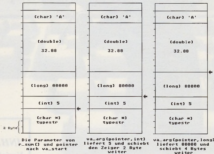
Der Stack und der Listenzeiger beim Aufruf von r_sum()
