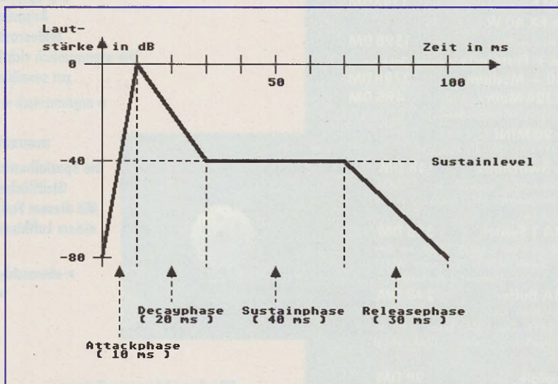
Abb. 2: Typischer Hüllkurvenverlauf am Beispiel der Amplitudenhüllkurve
