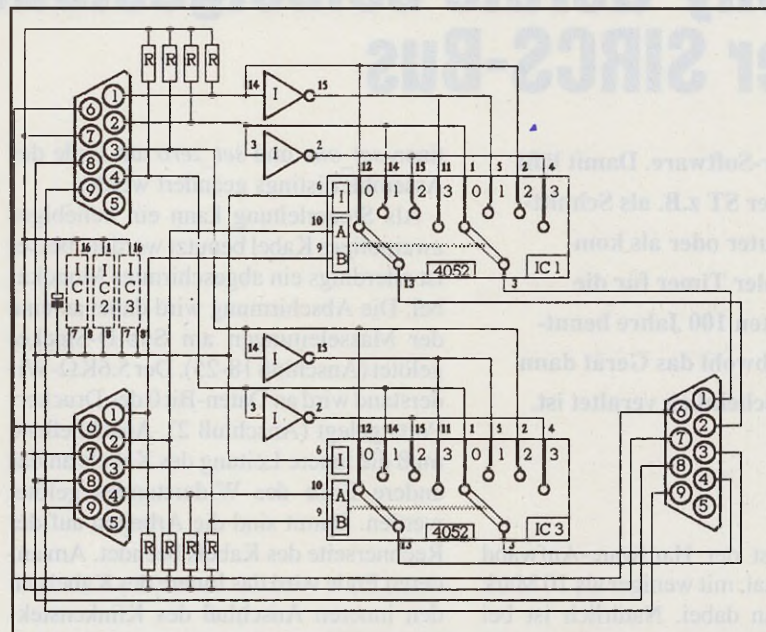
Das Schaltbild von Mausmixer
