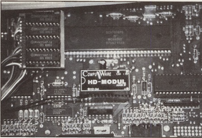
Mit nur drei Lötverbindungen wird das HD-Modul von Compu-Ware auf dem Floppycontroller befestigt.
