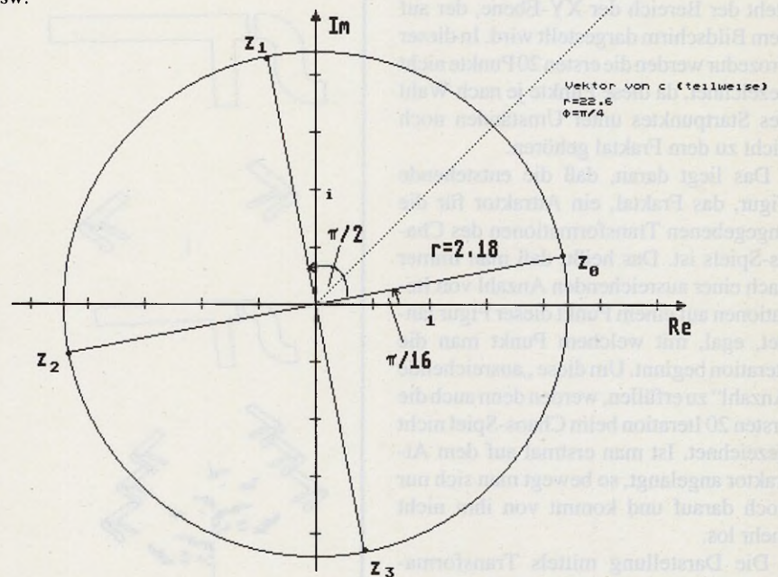
Die vier komplexen vierten Wurzeln von c = 16 + i*16
