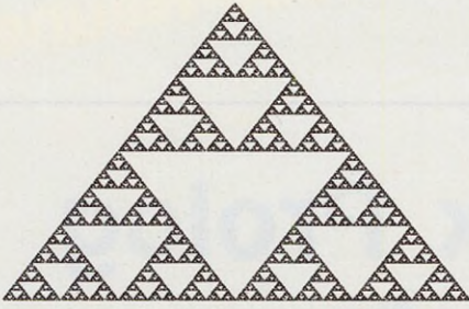
Bild 2: Hilfreich für das Chaos-Spiel - das Sierpinski-Dreieck
