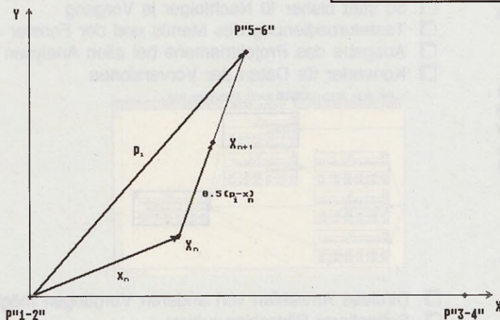
Bild 3: Konstruktion der Transformationsgleichung zum Sierpinski-Dreieck
