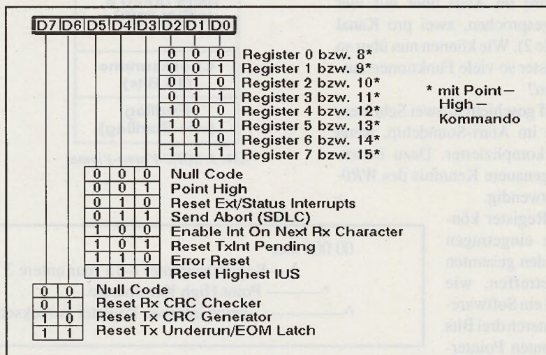
Abb. 5: Aufbau des WR0-Registers
