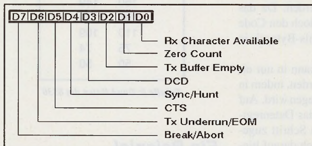
Abb. 7: Aufbau des RR0-Registers
