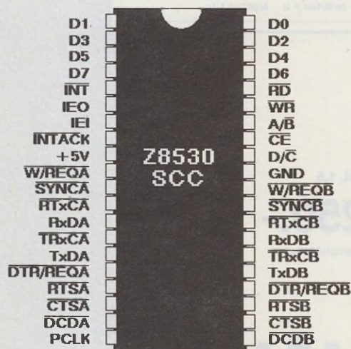
Abb. 2: Pinbelegung des SCC
