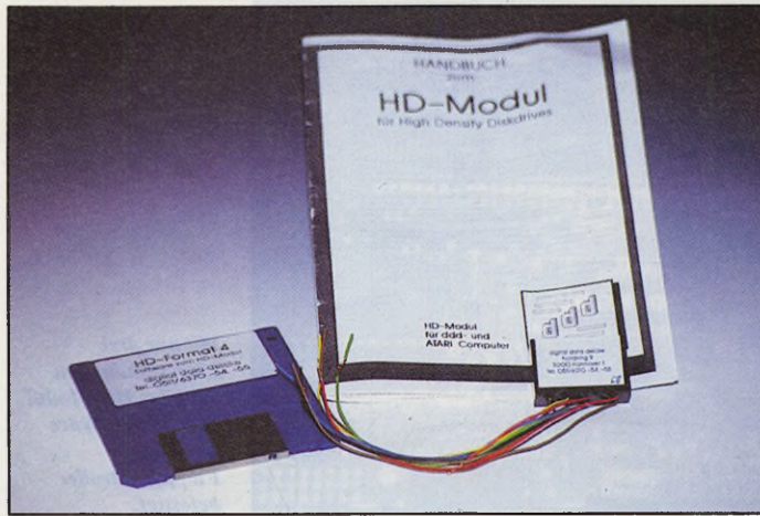
Viele Zuleitungen müssen zum Anschluß des HD-Moduls der Firma ddd gelötet werden.
