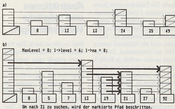
Bild 4a: „skip list“ mit Sprüngen 2 i
