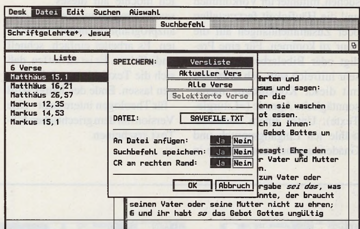
Bild 2: Im Suchbefehl-Fenster: Kombiniertes Suchbefehl mit Ergebnis
