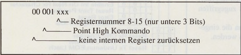
Abb. 4: Aufbau des Point-High-Kommandos
