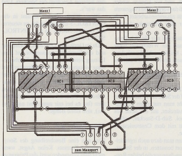
Der Verdrahtungsplan von Mausmixer
