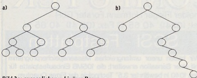
Bild 2a: ausgeglichener binärer Baum Bild 2b: degenerierter Baum
