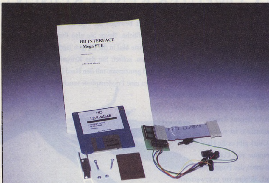
Den größten Lieferumfang bietet das HD-Interface für Mega STEs von Hard & Soft.
