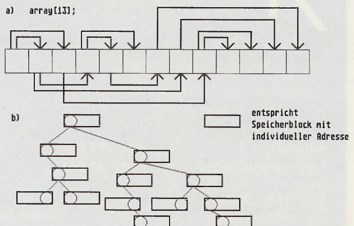
Bild 3a: Baum als array realisiert Bild 3b: dynamischer Baum realisiert
