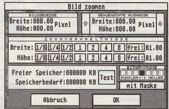
Bild 9: Mit dieser Dialogbox lassen sich die Bilder beliebig skalieren.
