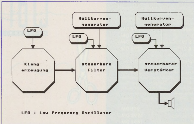
Abb. 1: Der grundlegende Aufbau von Synthesizern
